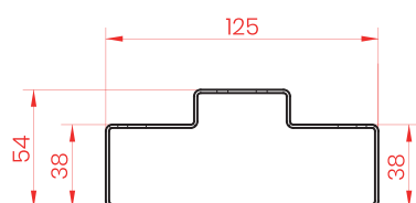
DOOR FRAME PROFILE
