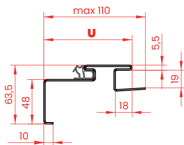
DOOR FRAME PROFILE
