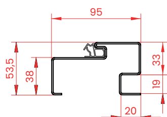
DOOR FRAME PROFILE
