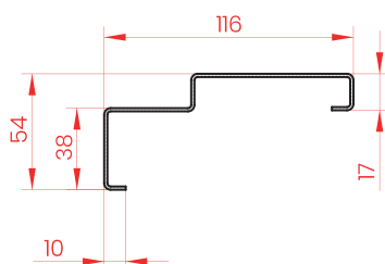
DOOR FRAME PROFILE
